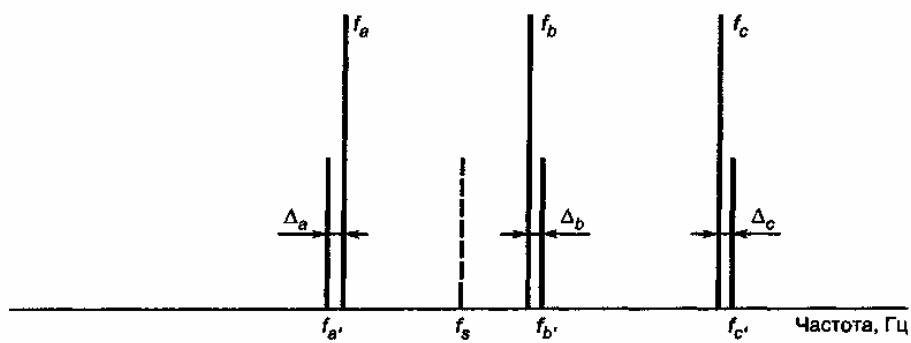
Рисунок Ж.1 — Примеры выбора частоты H_c
