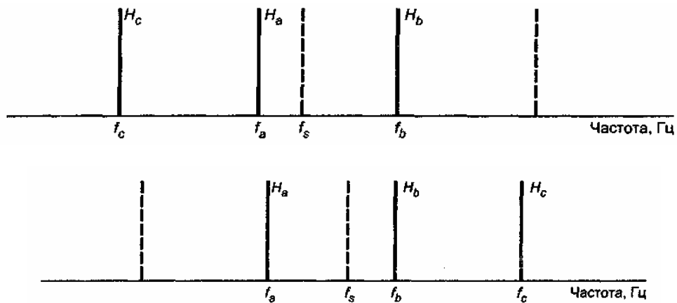
Рисунок Ж.1 — Примеры выбора частоты H_c
